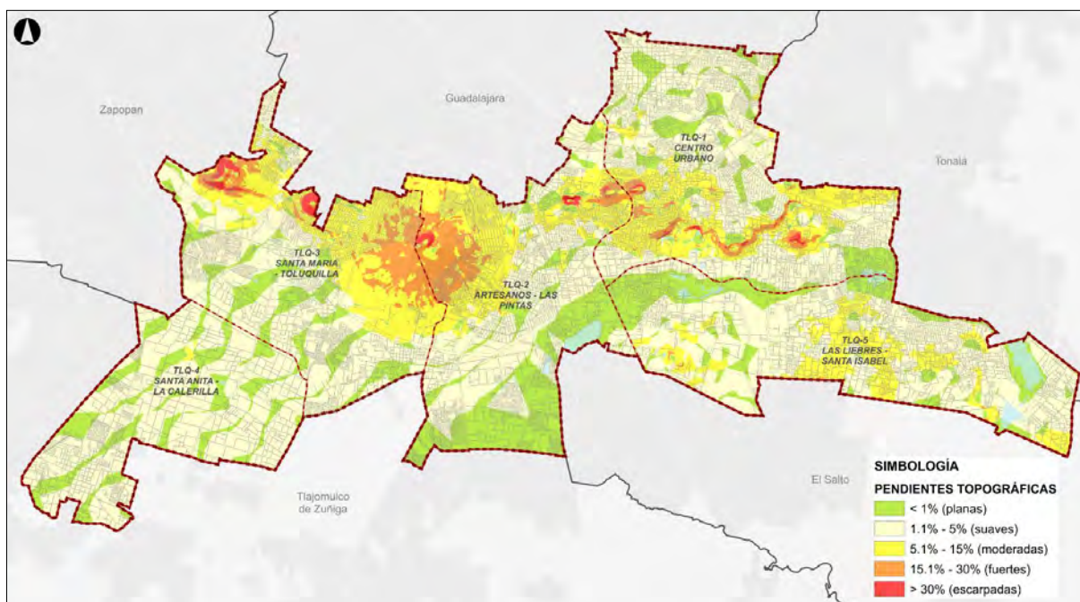
Figura 22. Pendientes topográficas del municipio de San Pedro Tlaquepaque.
