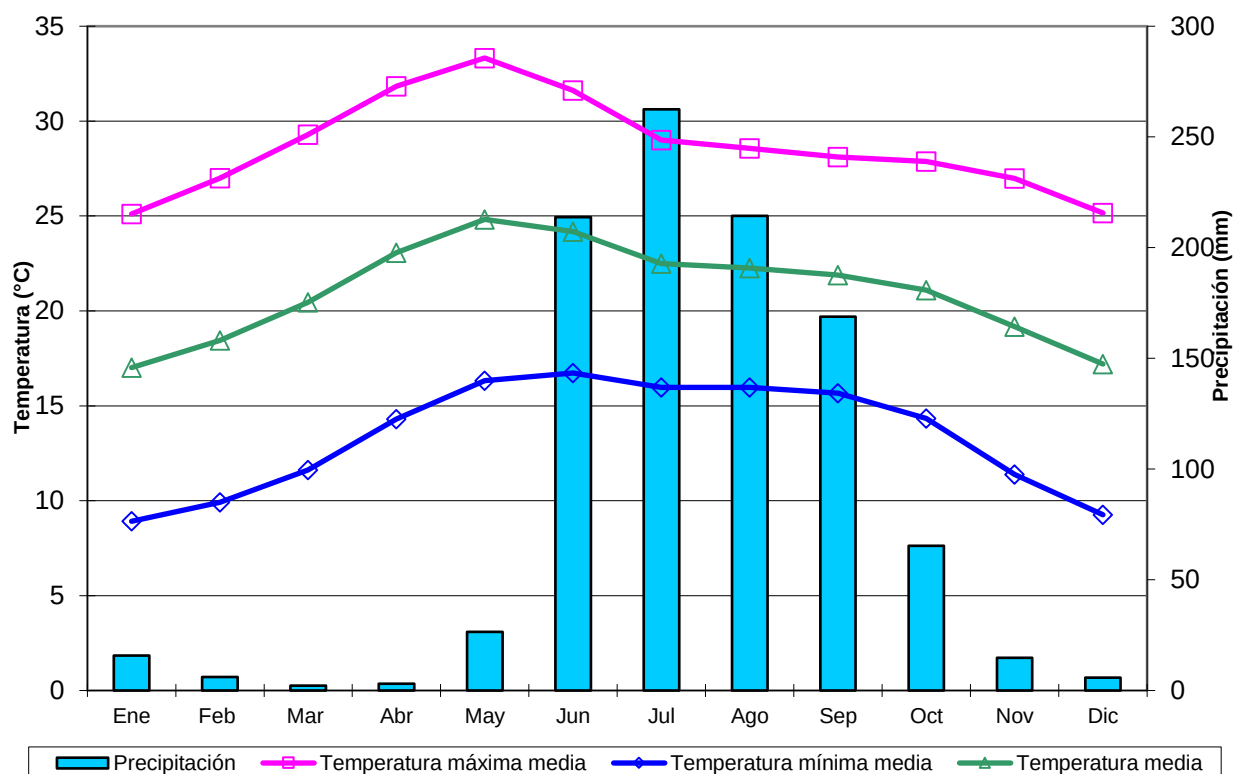
Figura 32. Patrón de variación mensual de precipitación y temperatura en Tlaquepaque.
