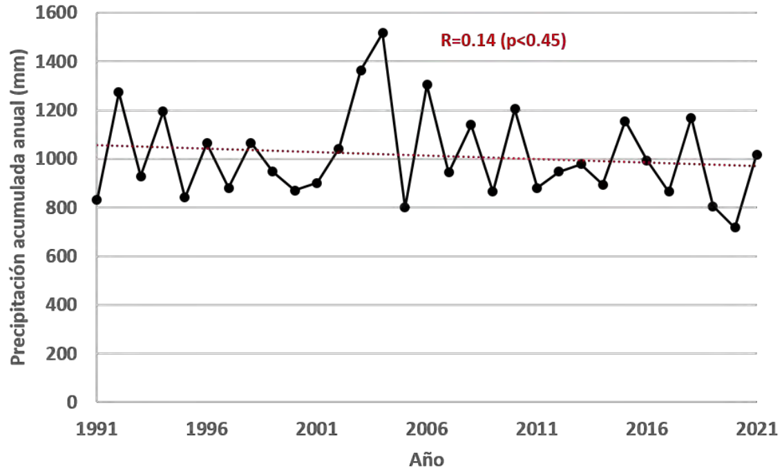
Figura 34. Tendencia de la precipitación en el Municipio de Tlaquepaque años 1991-2021.
