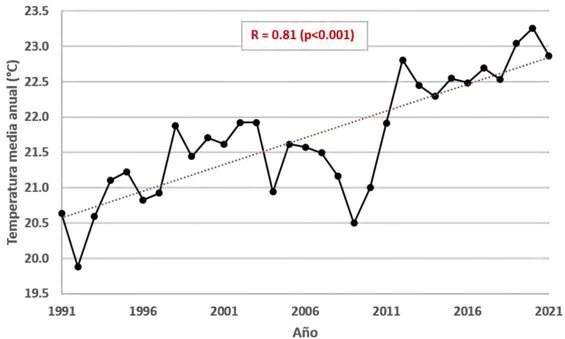
Figura 33. Tendencia de la temperatura en el Municipio de Tlaquepaque años 1991-2021.
