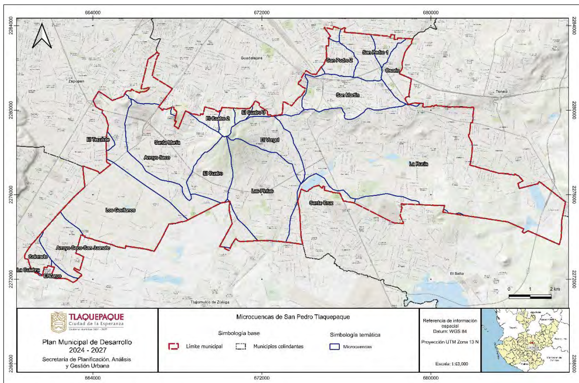
Figura 25. Distribución espacial de microcuencas del municipio de San Pedro Tlaquepaque.
