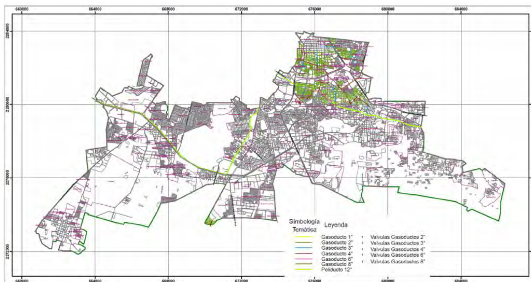
Figura 73. Red de ductos de gas natural en el municipio de San Pedro Tlaquepaque.
