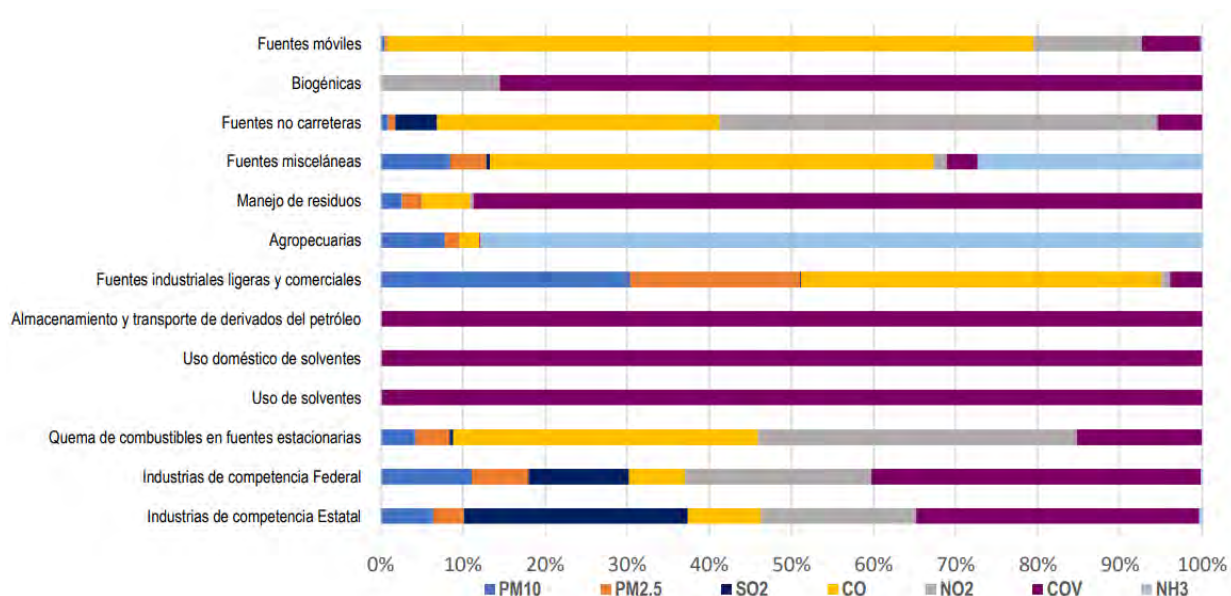
Figura 39. Fuentes emisoras y contribución porcentual para la emisión de contaminantes criterio en el Área Metropolitana de Guadalajara.
