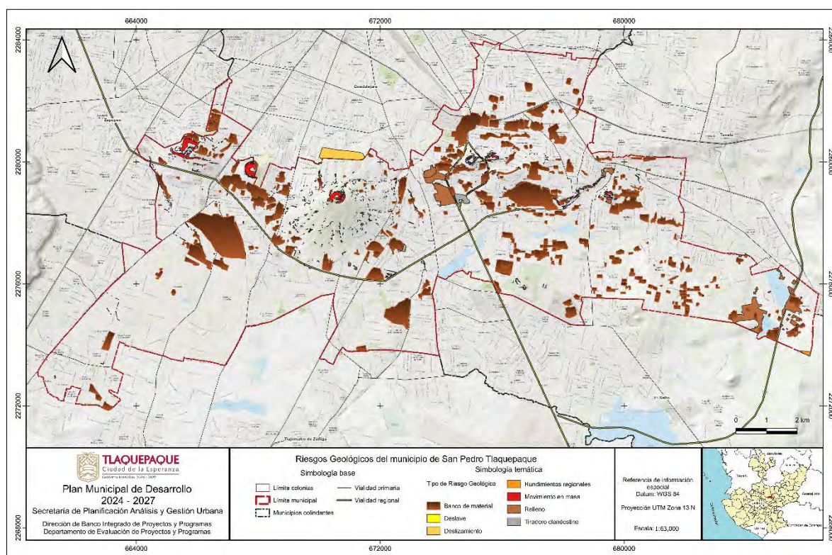
Figura 71. Riesgos geológicos del municipio de San Pedro Tlaquepaque.
