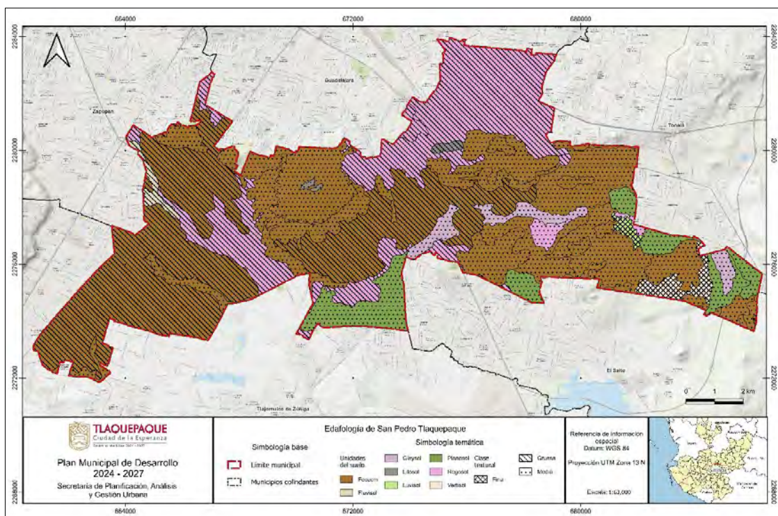
Figura 24. Distribución espacial de tipos de suelo de San Pedro Tlaquepaque. Fuente: Elaboración propia con base en conjunto de datos vectoriales edafológicos del IIEG.
