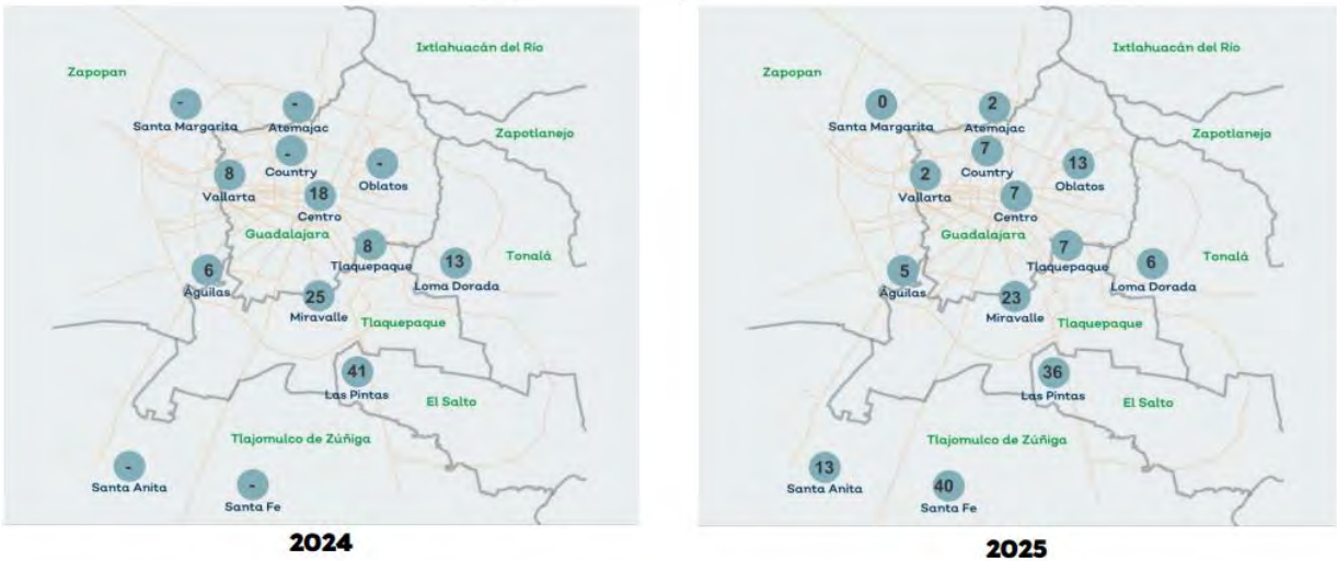
Figura 37. Número de días con mala calidad del aire en el Área Metropolitana de Guadalajara en los años 2024 y 2025 (avance).
