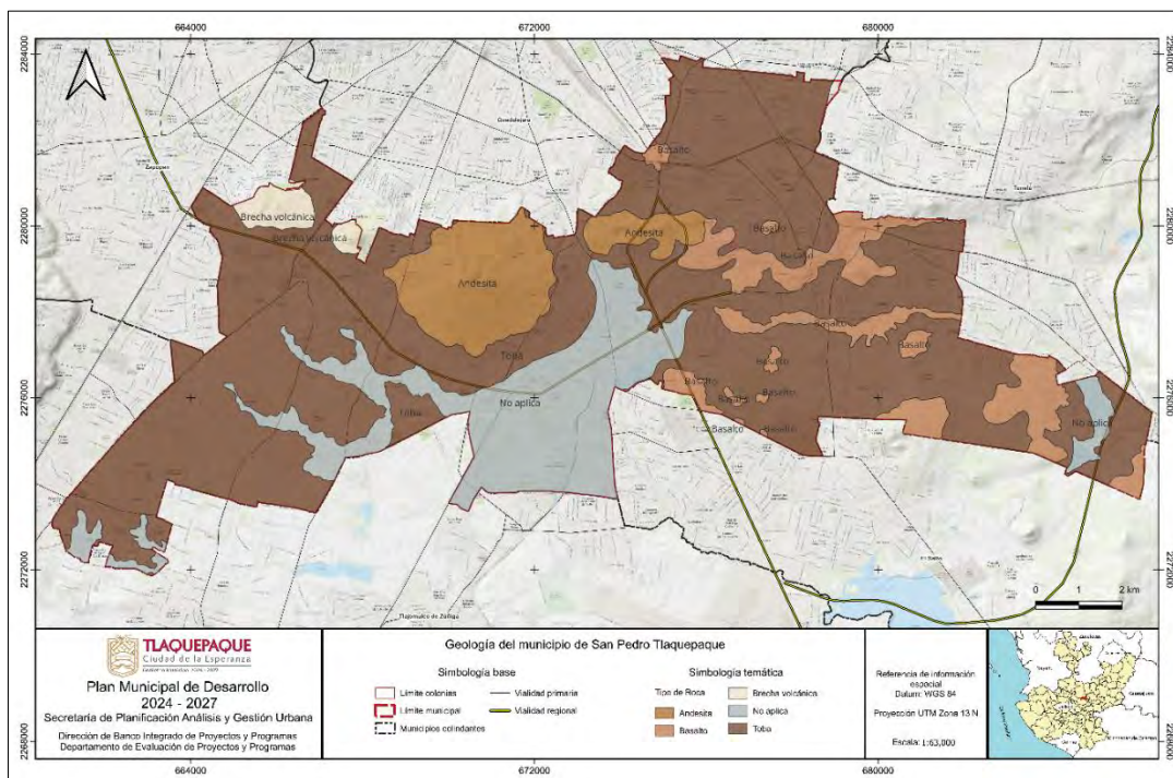
Figura 23. Geología del municipio de San Pedro Tlaquepaque.
