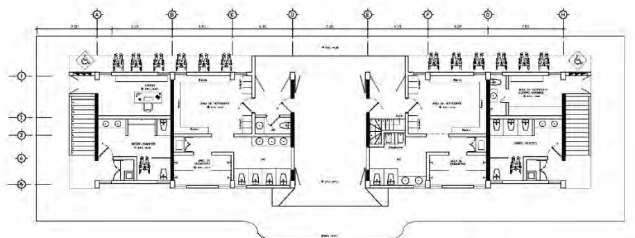
PLANTA ARQUITECTÓNICA BAJA
